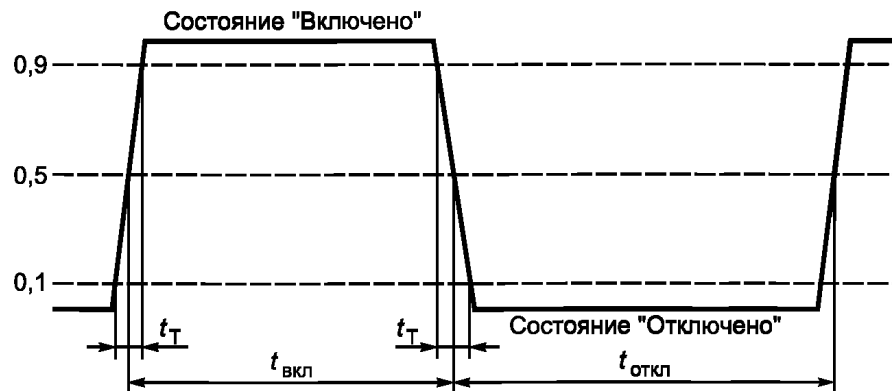
Рисунок D.1 — Испытательная схема испытательного выходного устройства
