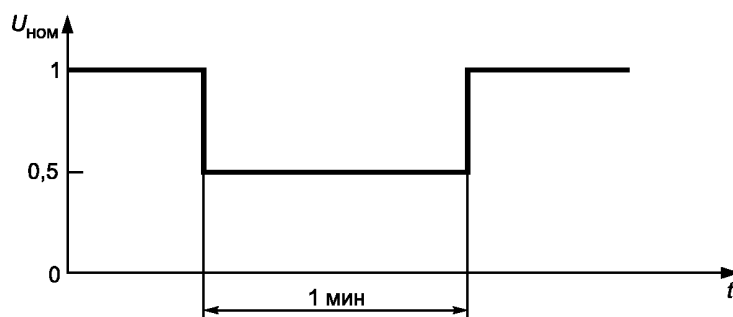
Рисунок В.3 — Провалы напряжения \Delta U = 50\%
